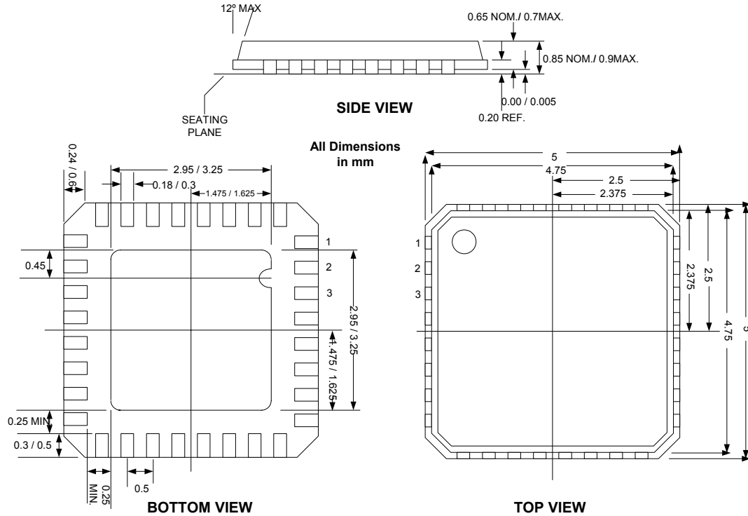
32 pin QFN
