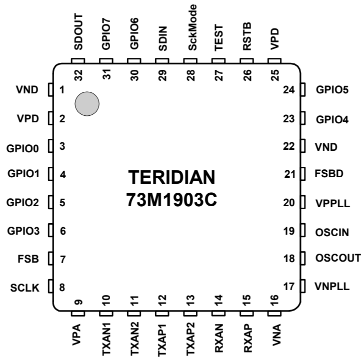
73M1903C QFN 32
